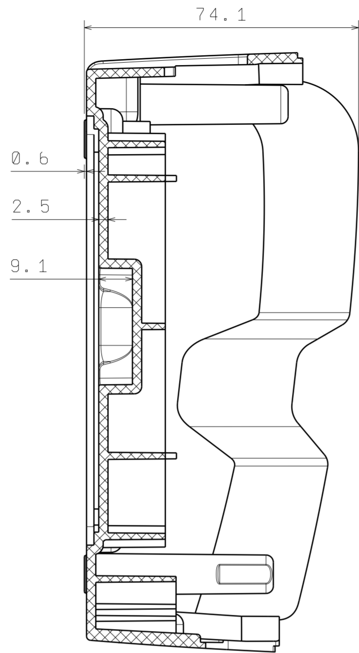
Section view A-A Scale: 1:1
