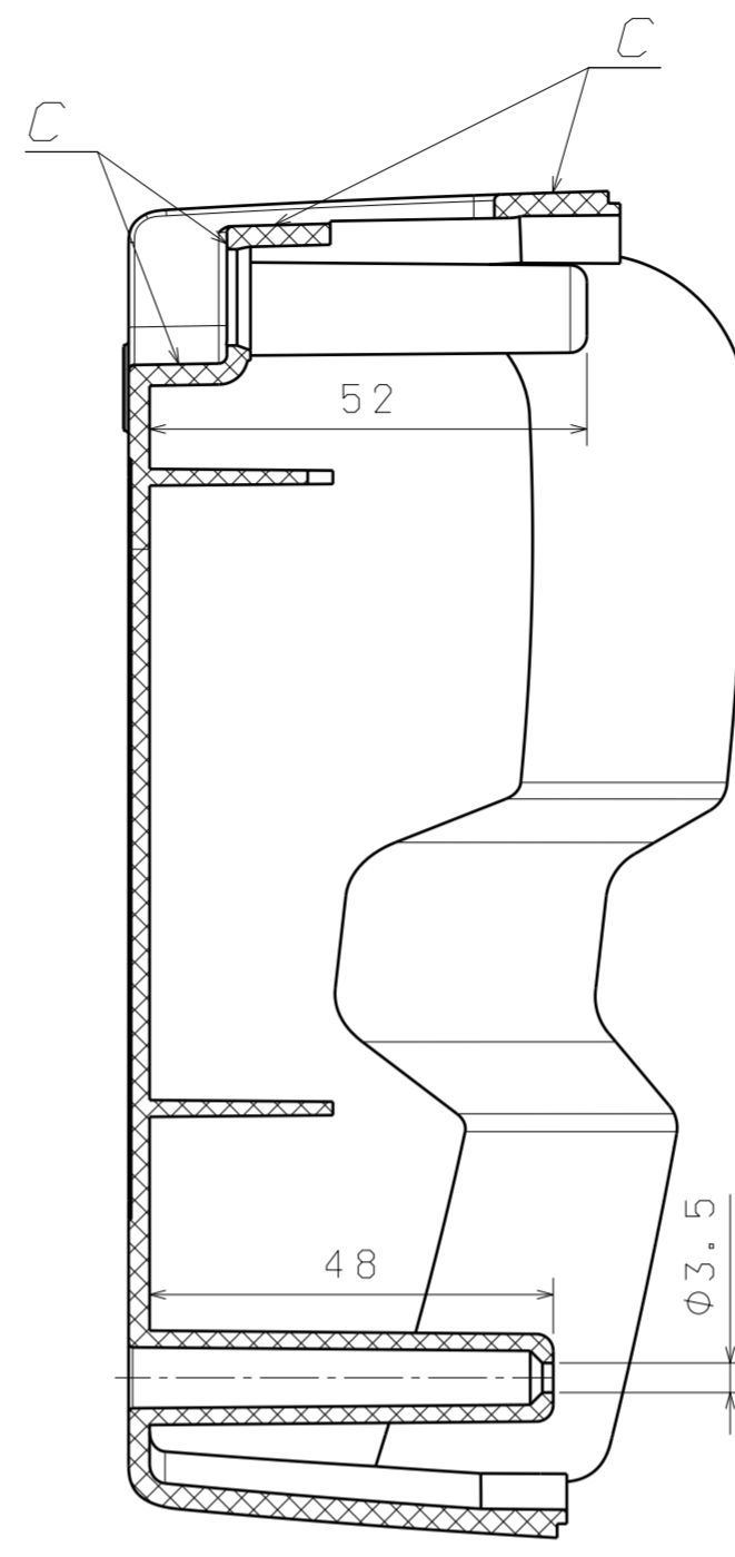
Section view B-B Scale: 1:1
